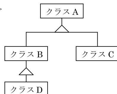
<クラスの継承図>
